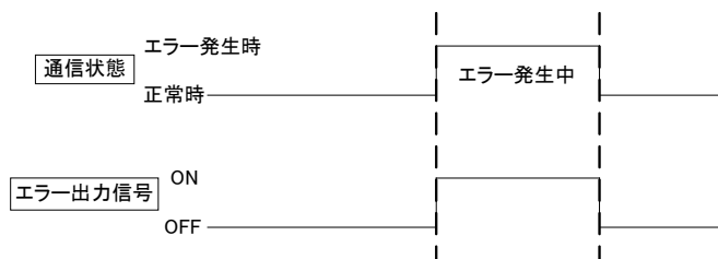
エラー出力信号 a 接点
