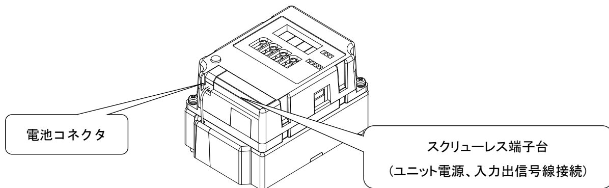
パルスカウント子局の配線
