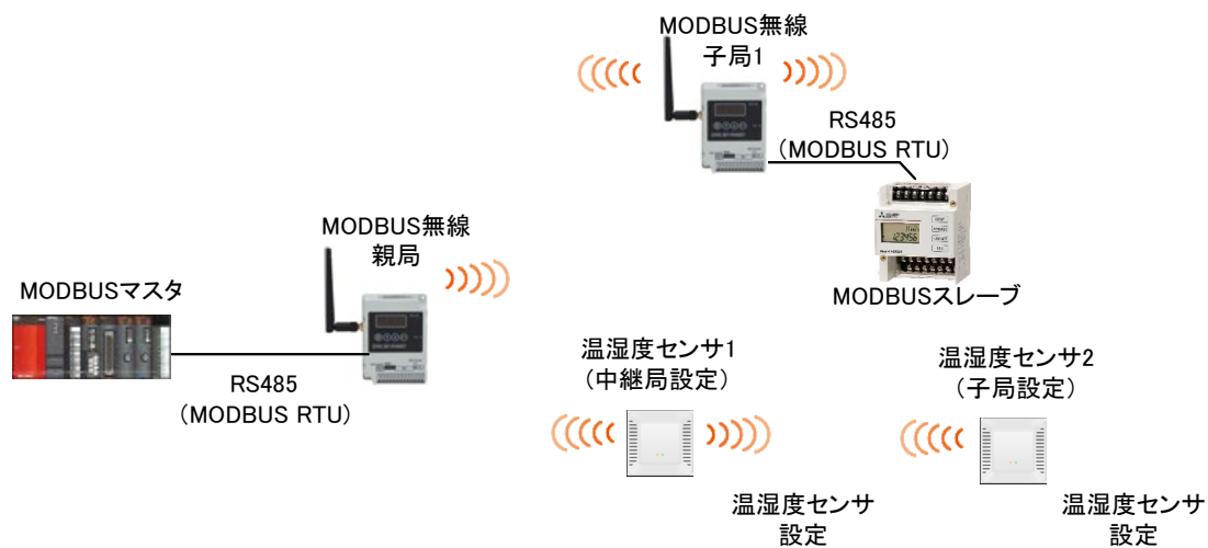
温湿度センサ接続
