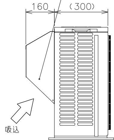
吸込フード（後） （AGJT-13B）
