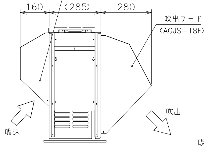
吸込フード（後） （AGJS-18B）
