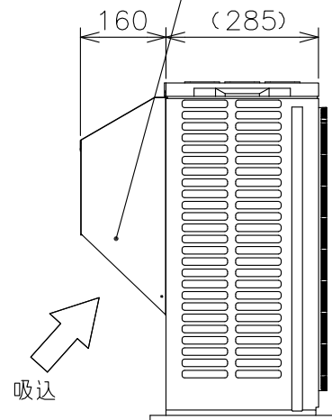
吸込フード（後） （AGJT-18B）
