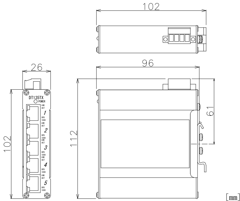
图 6. 1 外形规格
