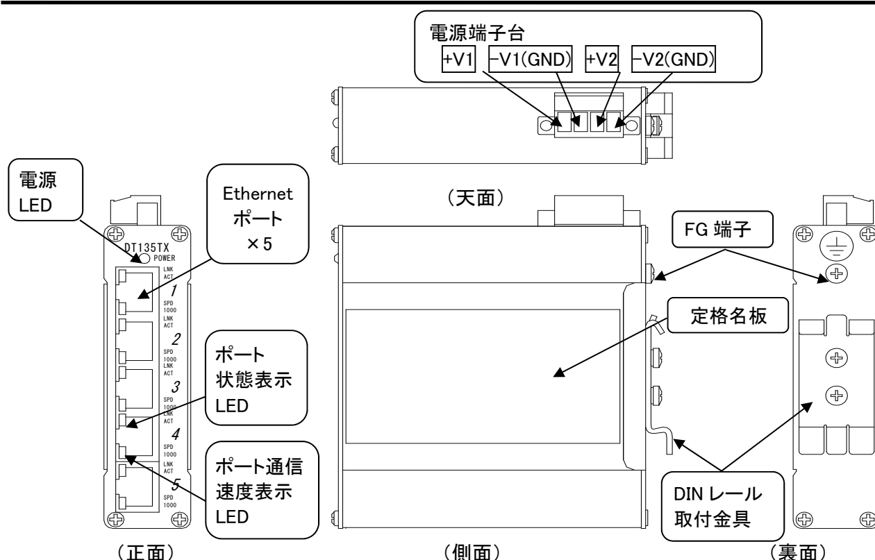
図 4.1 各部の名称
