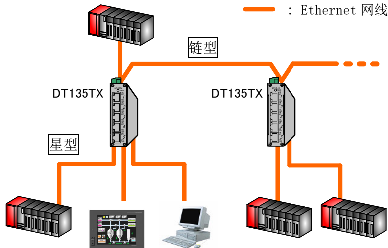
图 2.1 连接范例
