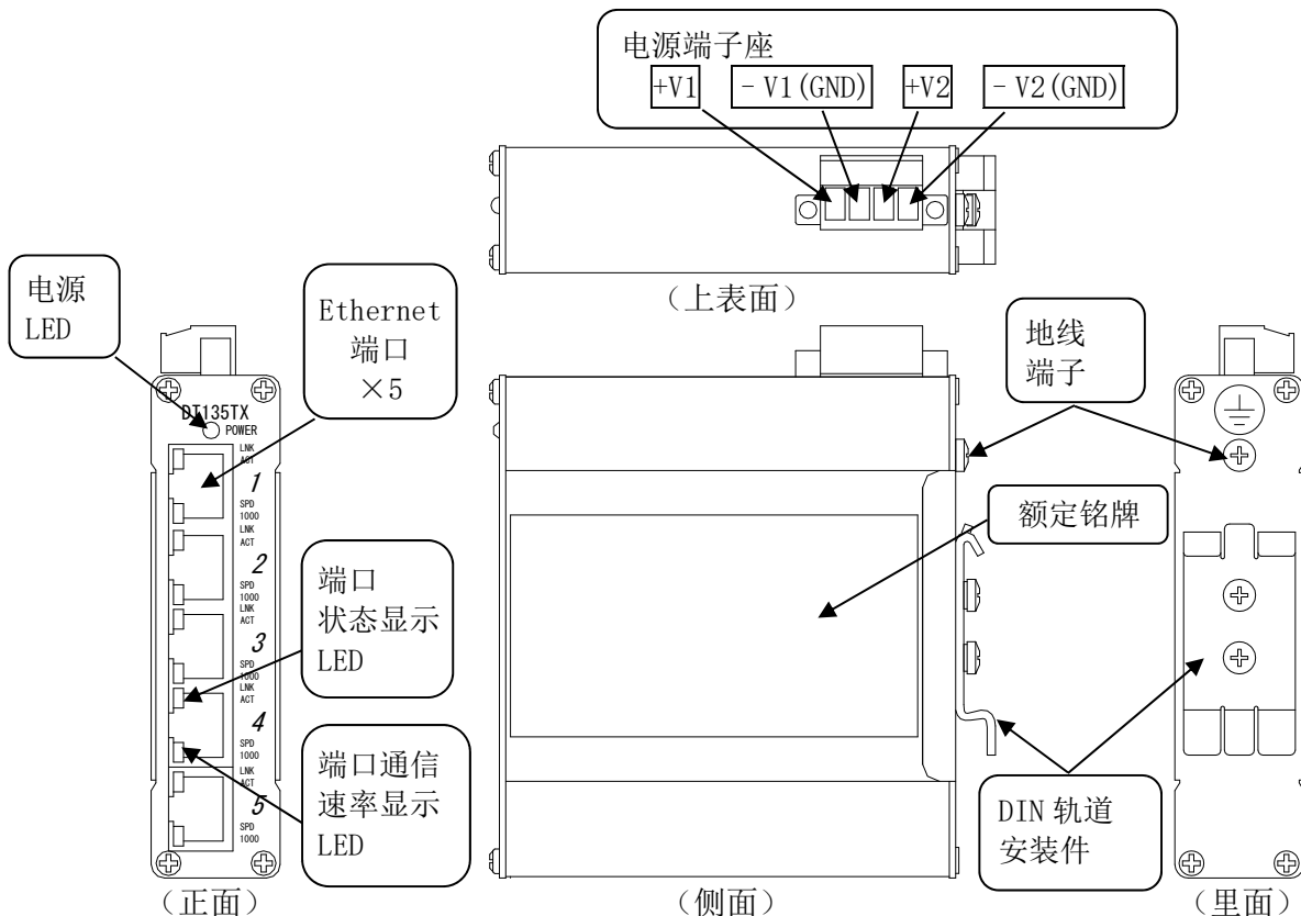
图 4.1 各部分名称
