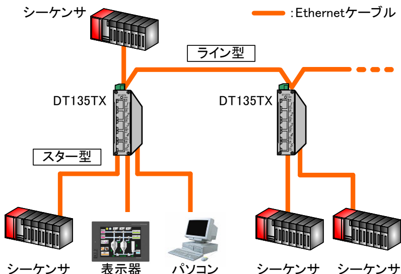
図 2.1 接続例
