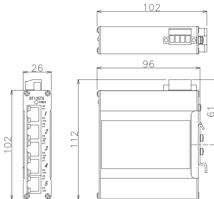
図 6.1 外形寸法
