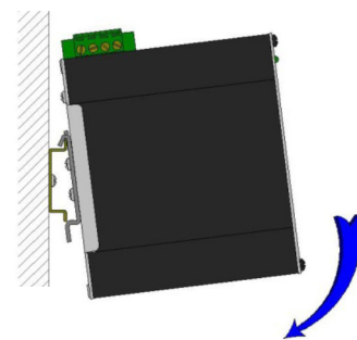
图 5.1 安装方法
