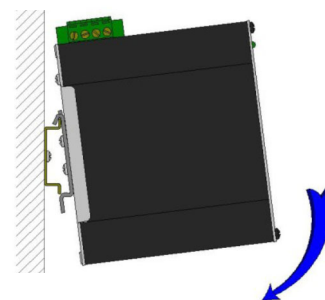
図 5. 1 取付方法
