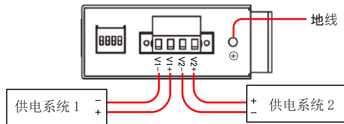
图 5.2 电源接线（冗余电源）
