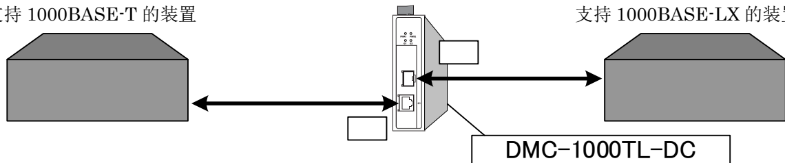
图 2.2 1000BASE-T↔LX 转换连接示例
