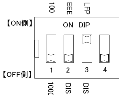
図 5. 1 DIP スイッチ設定
