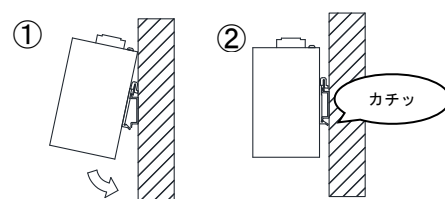
図 5.3 取付け方法
