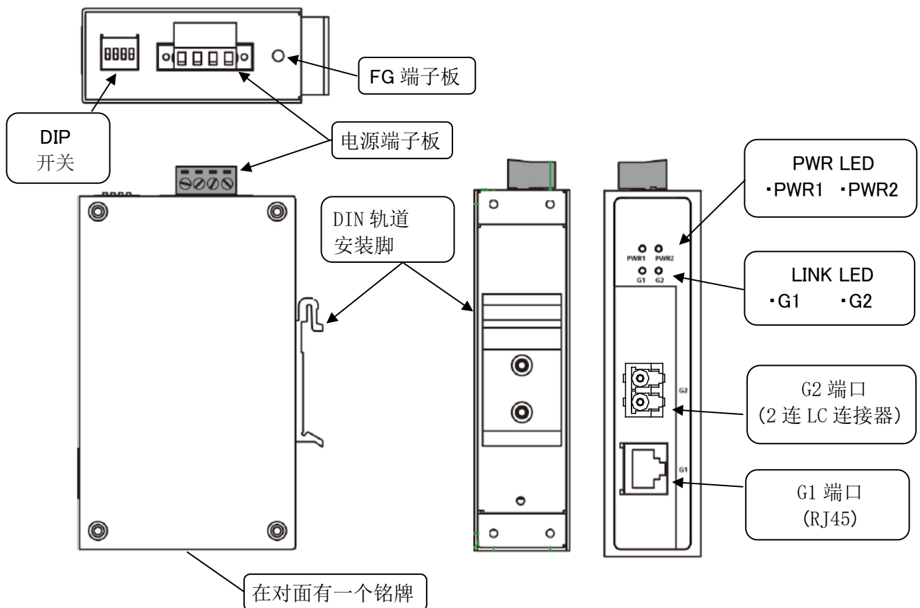
图 4.1 部件名称
