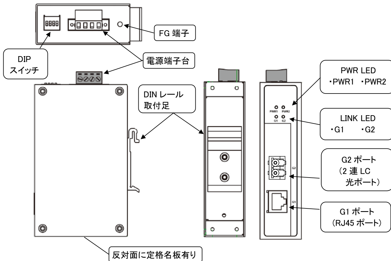
図 4. 1 各部の名称
