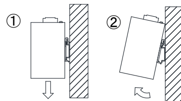
図 5.4 取外し方法
