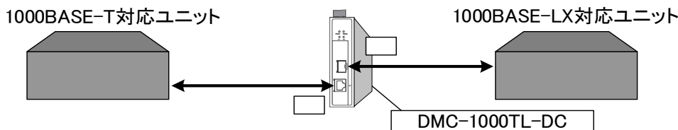
図 2. 2 1000BASE-T⇔LX 変換接続例
