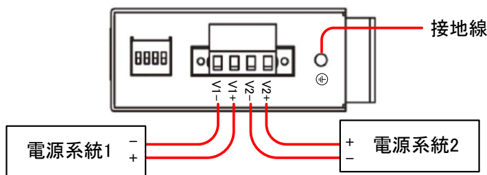
図 5. 2 電源配線 (冗長電源)
