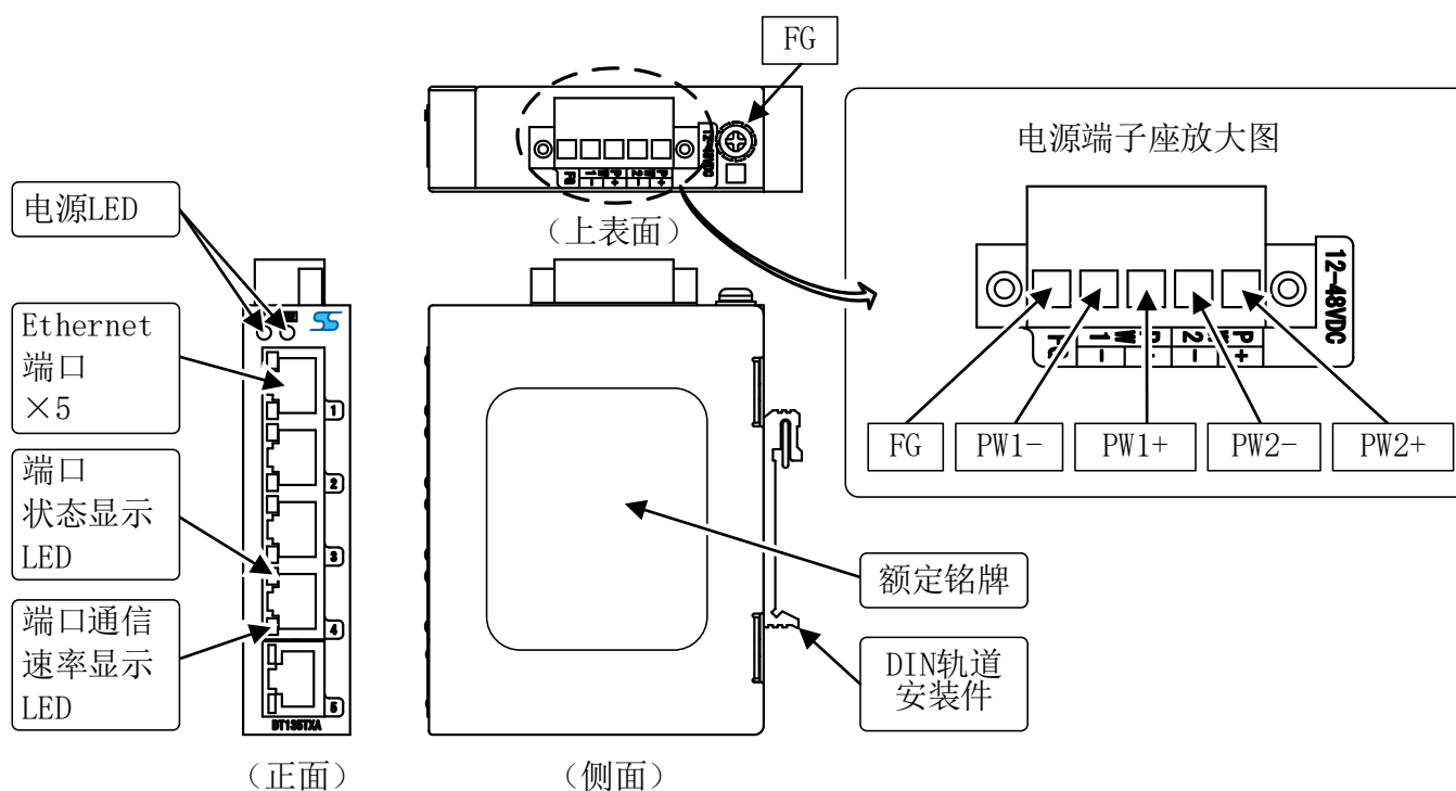
图 4.1 各部分名称
