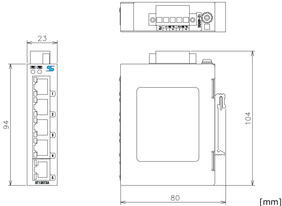
図 6. 1 外形寸法
