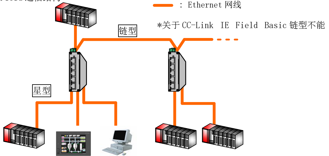
图 2.1 连接范例
