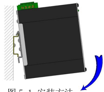
图 5.1 安装方法
