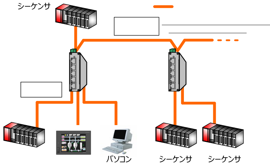
図 2. 1 接続例
