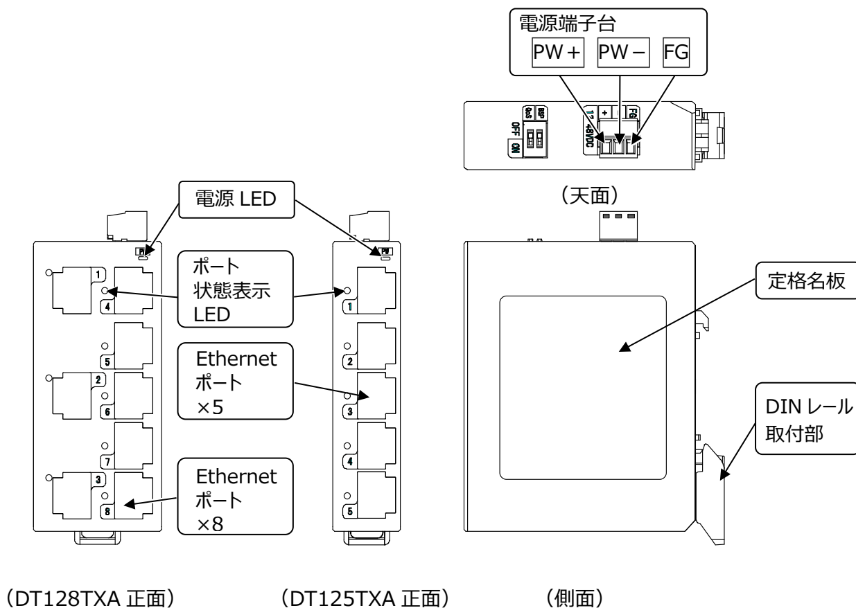
図 4. 1 各部の名称
