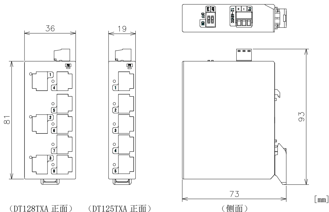
图 6. 1 外形规格
