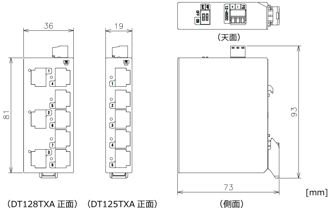
図 6. 1 外形寸法
