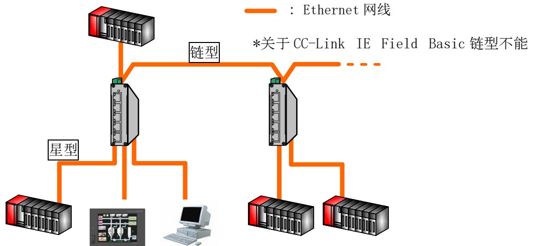
图 2.1 连接范例
