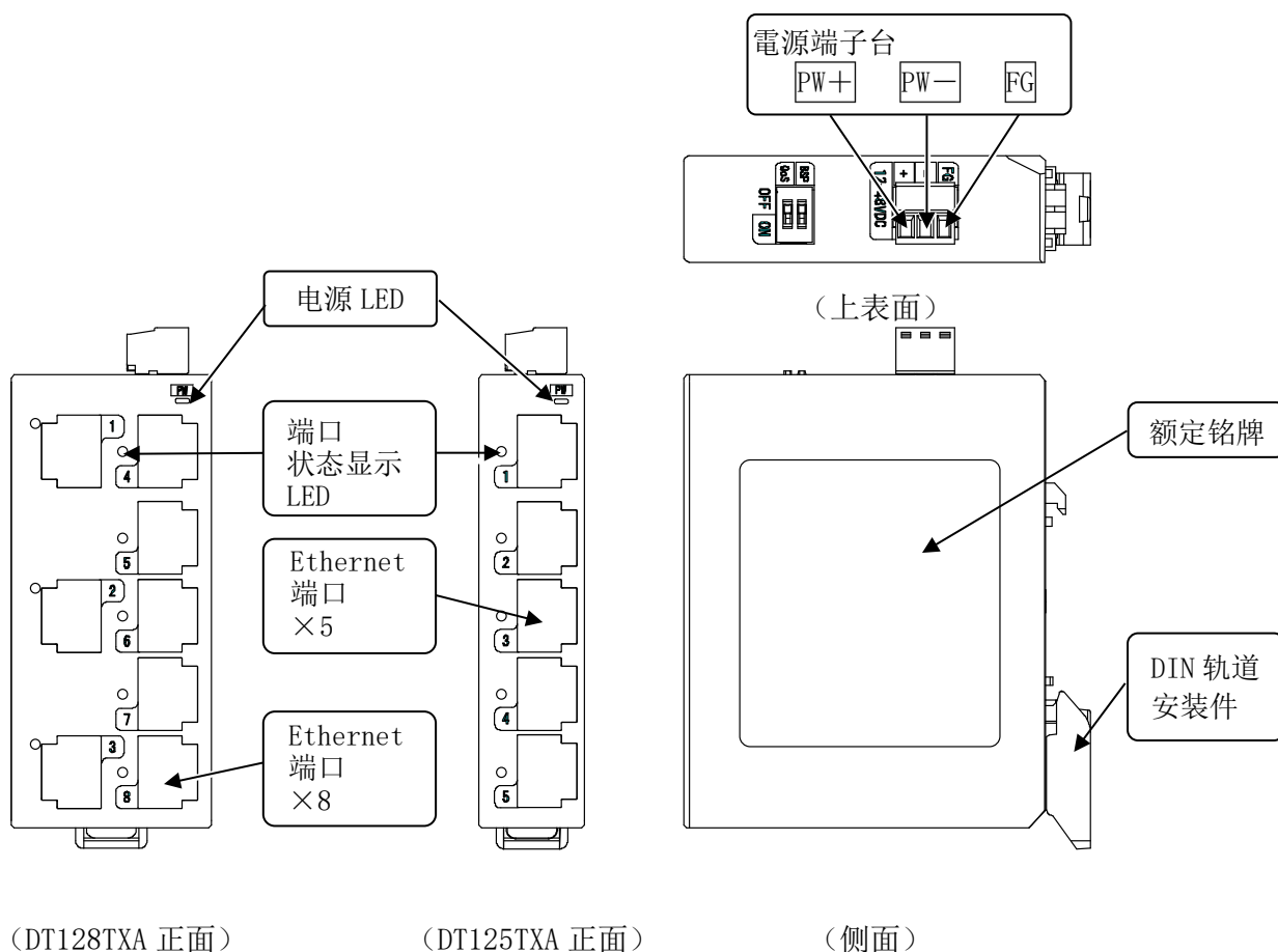
图 4.1 各部分名称
