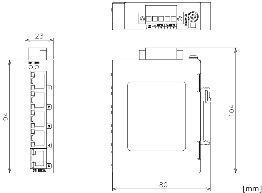
図 6. 1 外形寸法
