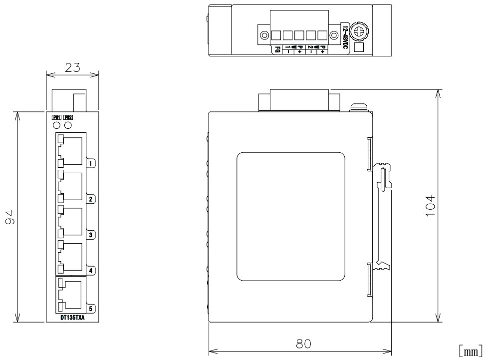
图 6. 1 外形规格
