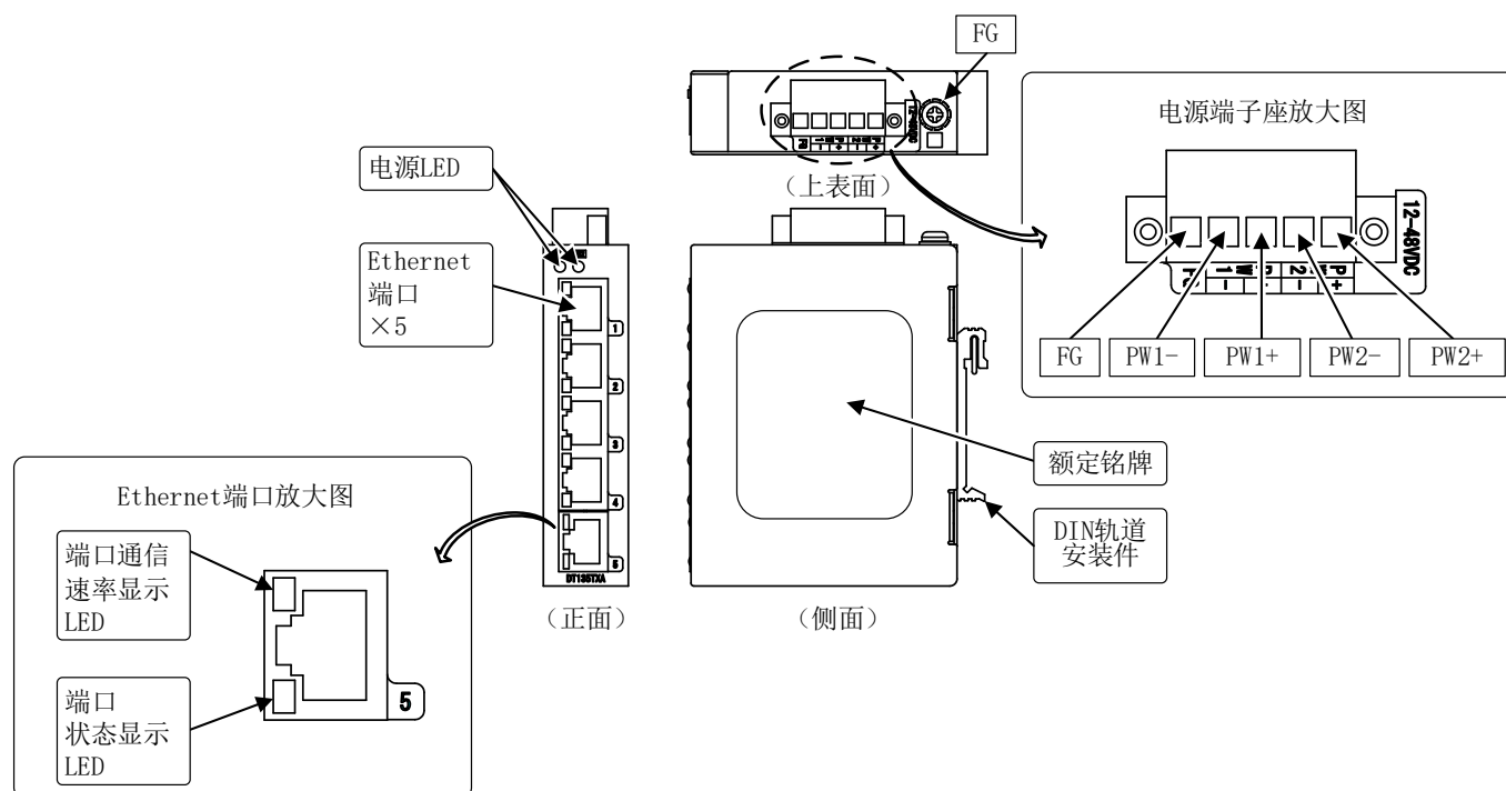
图 4.1 各部分名称
