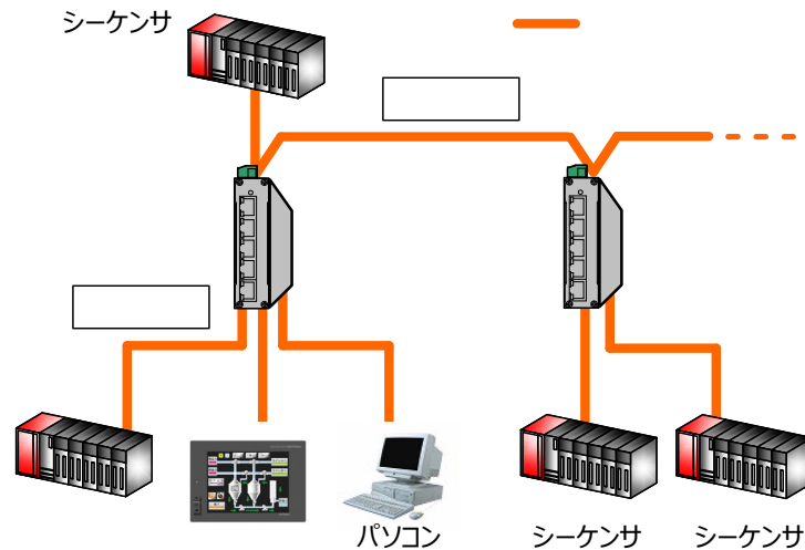
図 2. 1 接続例
