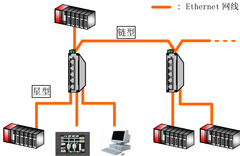
图 2.1 连接范例
