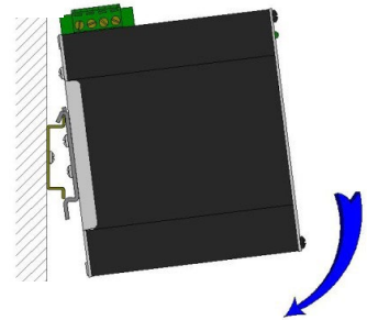
图 5.1 安装方法
