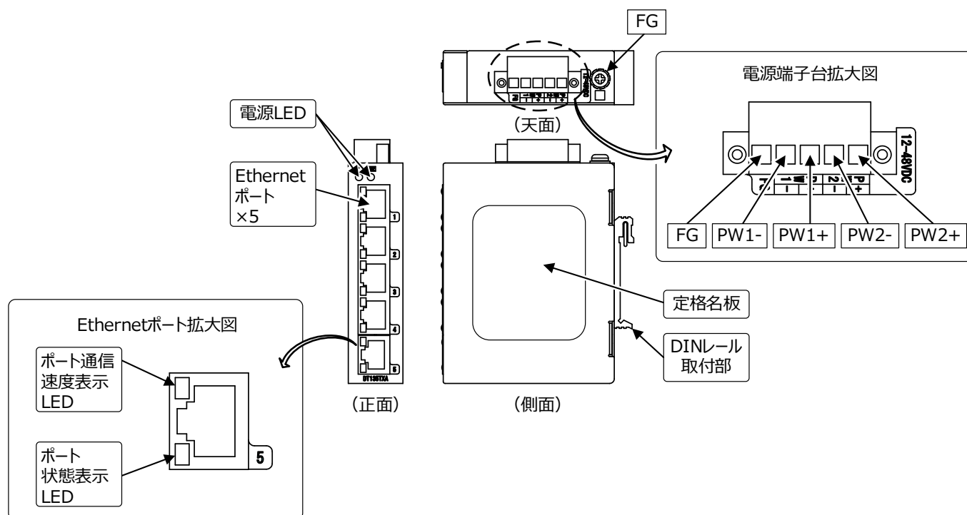
図 4. 1 各部の名称
