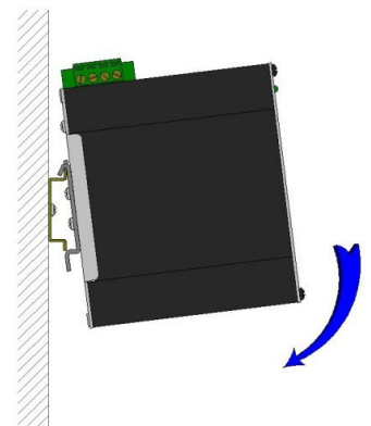
図 5. 1 取付方
