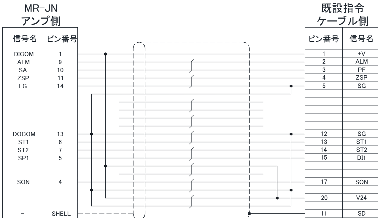
SC-CAJNCTC03M-S結線図
