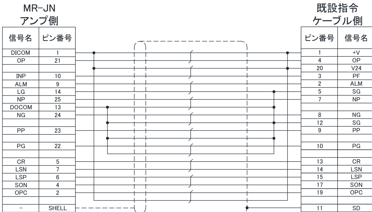
SC-CAJNCTC03M-P結線図
