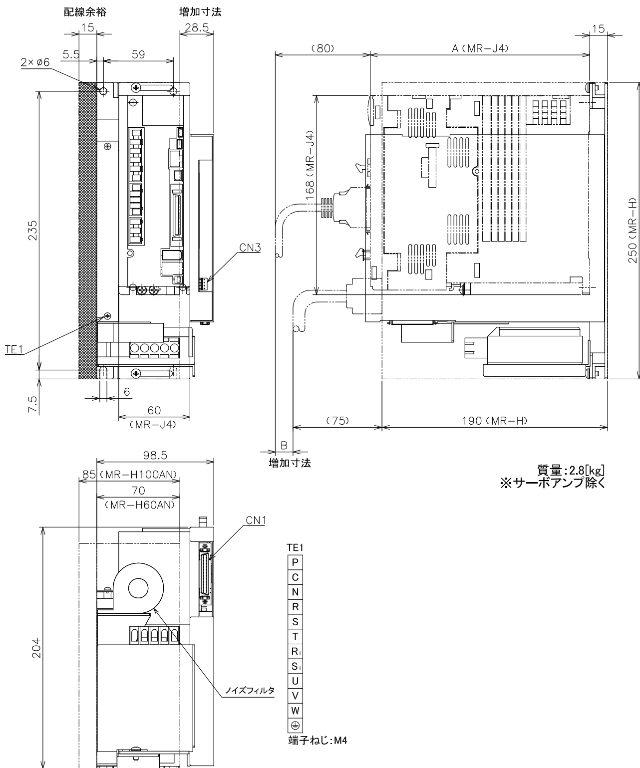
変化寸法表
