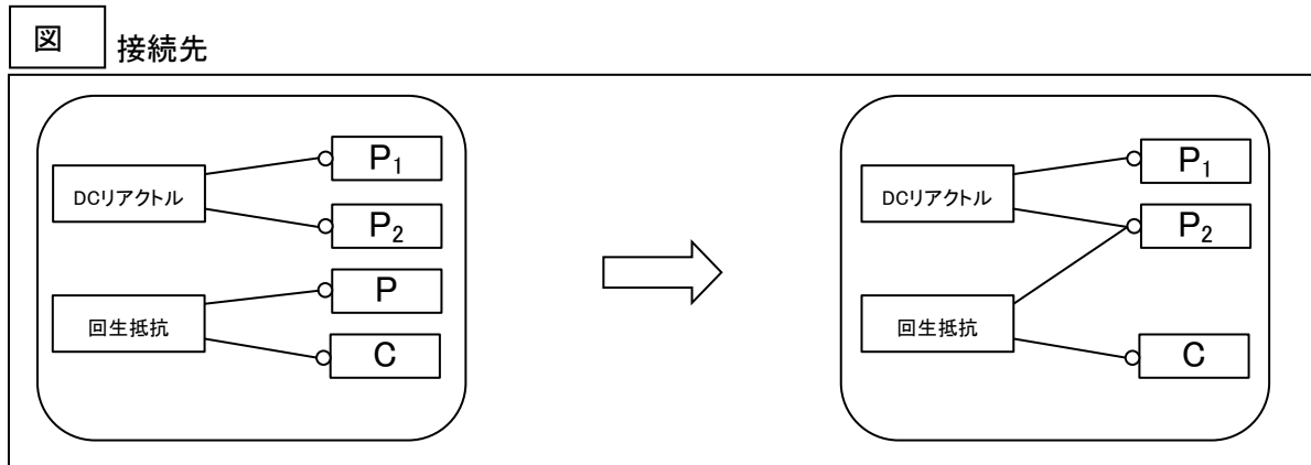
J2S コンバータユニットの既設配線
