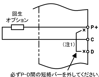
回生オプションの接続 (SC-J2SBJ4KT5Kの場合)
