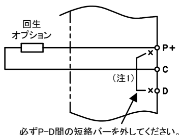
回生オプションの接続 (SC-J2S(CP)J4KT5Kの場合)
