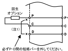
回生オプションの接続 (SC-J2SBJ4KT02K~1Kの場合)
