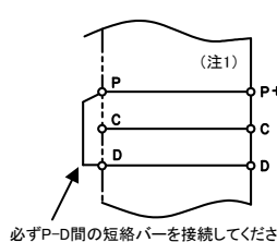
回生オプションがない場合の接続 (SC-J2SBJ4KT02K~1Kの場合)
