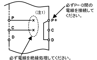
(SC-J2S(CP) J4KT3Kの場合)
