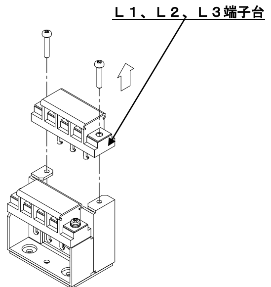
② バッテリーありの場合 (絶対位置検出システムの場合)
