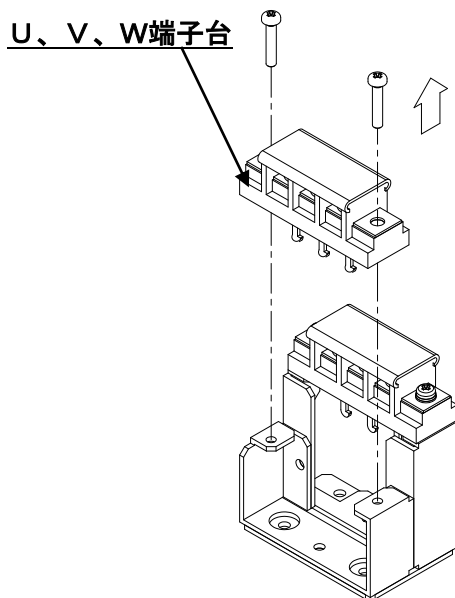
① バッテリーなしの場合 (インクリメンタルシステムの場合)
