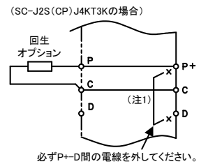
(SC-J2S(CP) J4KT3Kの場合)
