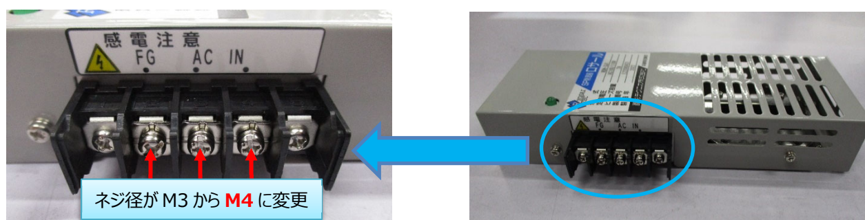
図 1 外観 (RDH-3J1)
