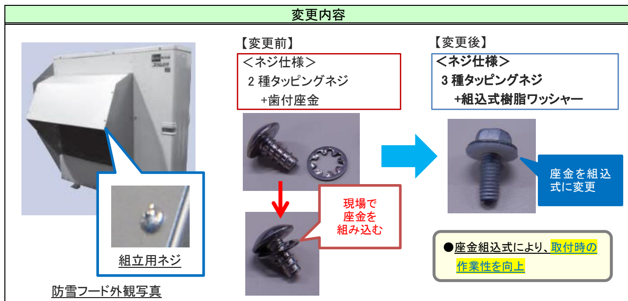
図 1. 組立用ネジ変更
