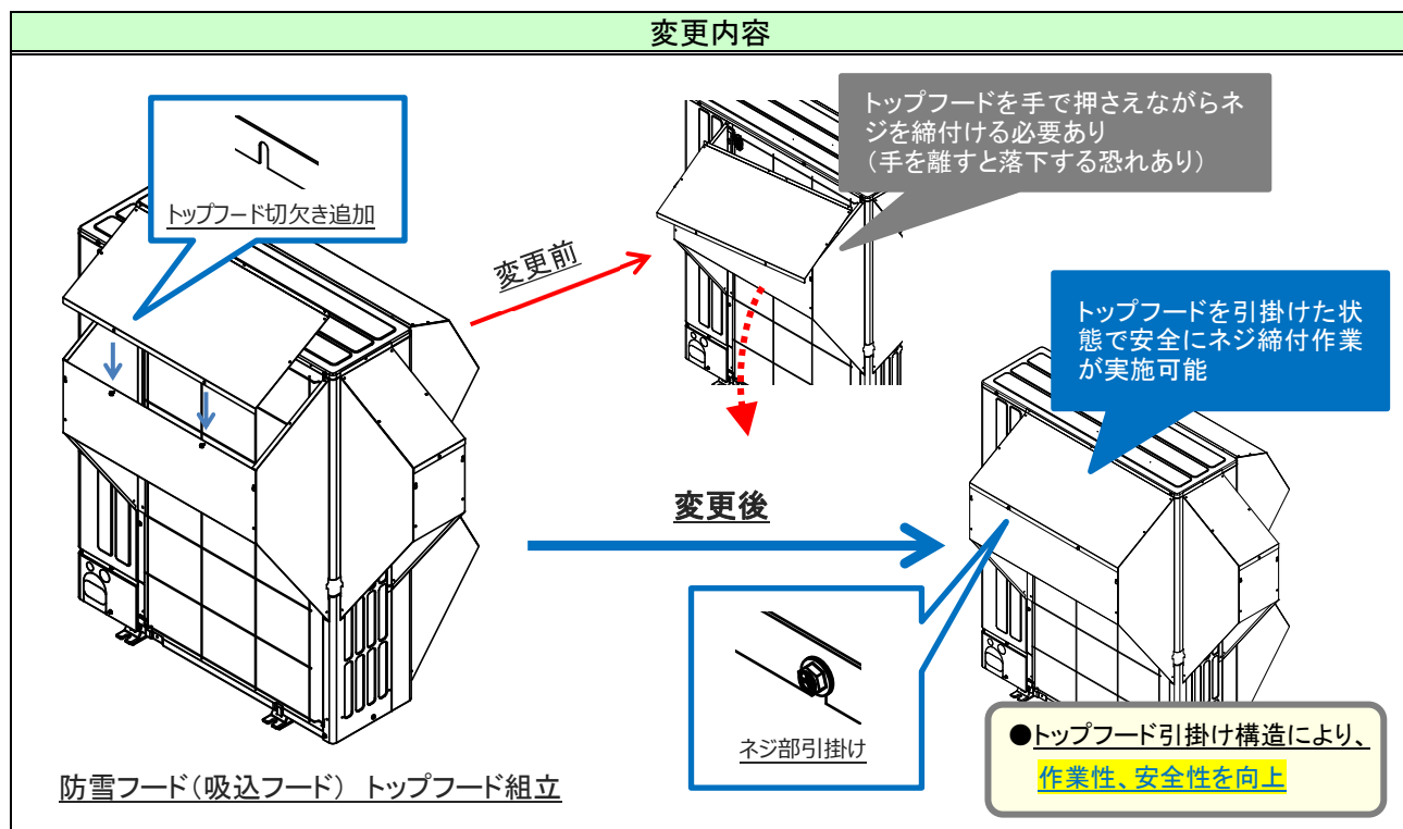
図 2. トップフード引掛け用切欠き追加
