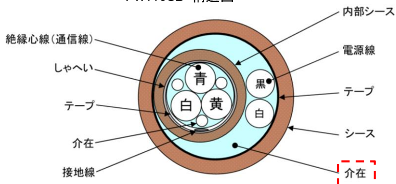
PW110SB 構造図
