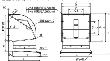
■給排気形 防火タイプ(70, 80cm)
