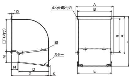
■給排気形 標準タイプ(20~60cm)
