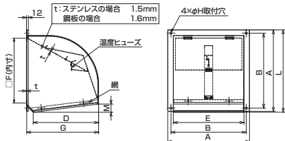
■排気形 防火タイプ(20~60cm)
