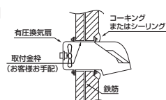
断面図
