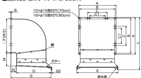
■給排気形 標準タイプ(70, 80cm)
