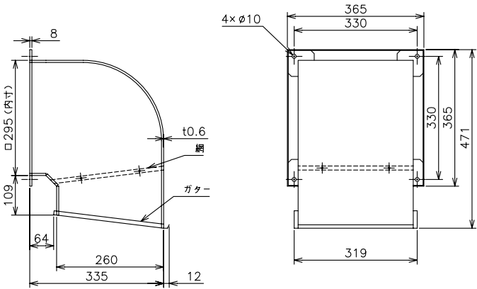
網部分詳細
