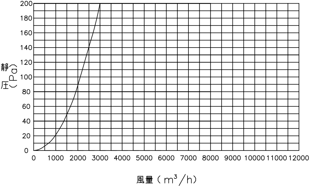
標準タイプ（排気）
