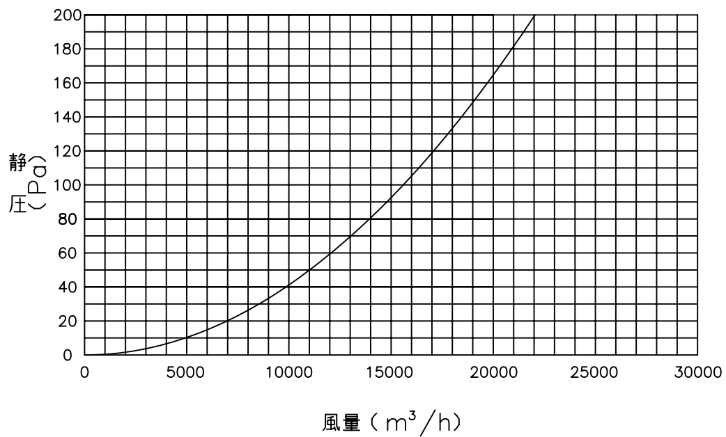
防火タイプ（給気）
