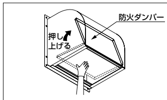
③防火ダンパーを下方から押し上げます。
