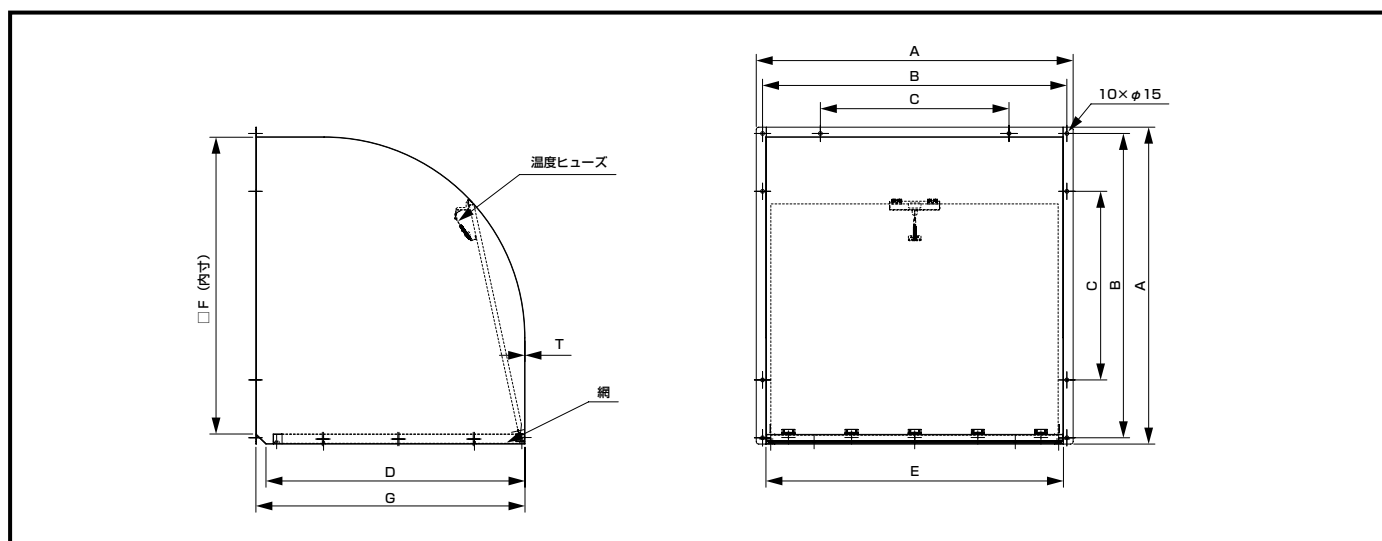
外形寸法表
