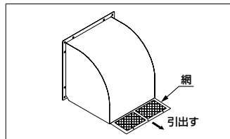
②フード正面側から網を引出す。
