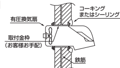
断面図
