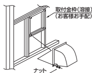
取付図 (壁面埋込)
