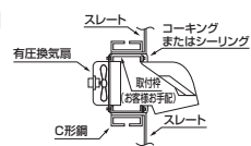
断面図
