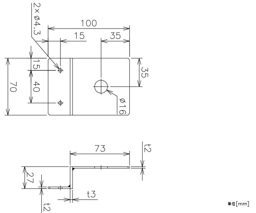
アンテナ固定具 (材質: 樹脂)
