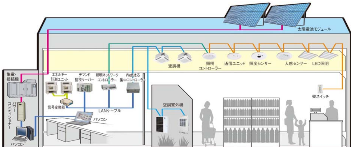
「SA1-MICO」のシステム構成例
