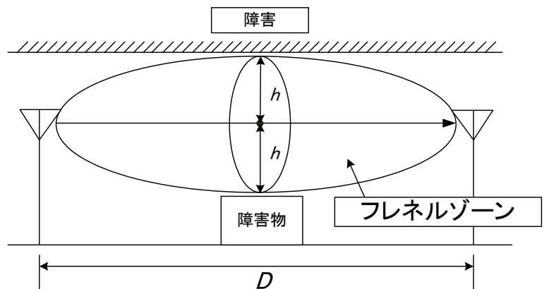
図7: フレネルゾーン
